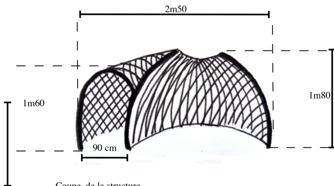
Coupe de la structure
